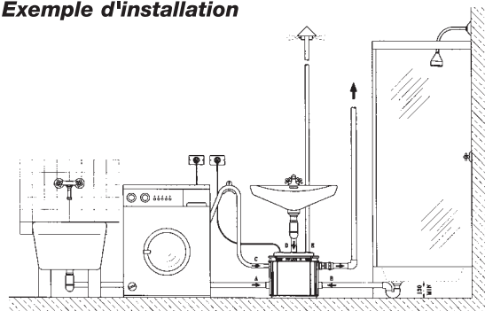
Exemple d'installation
